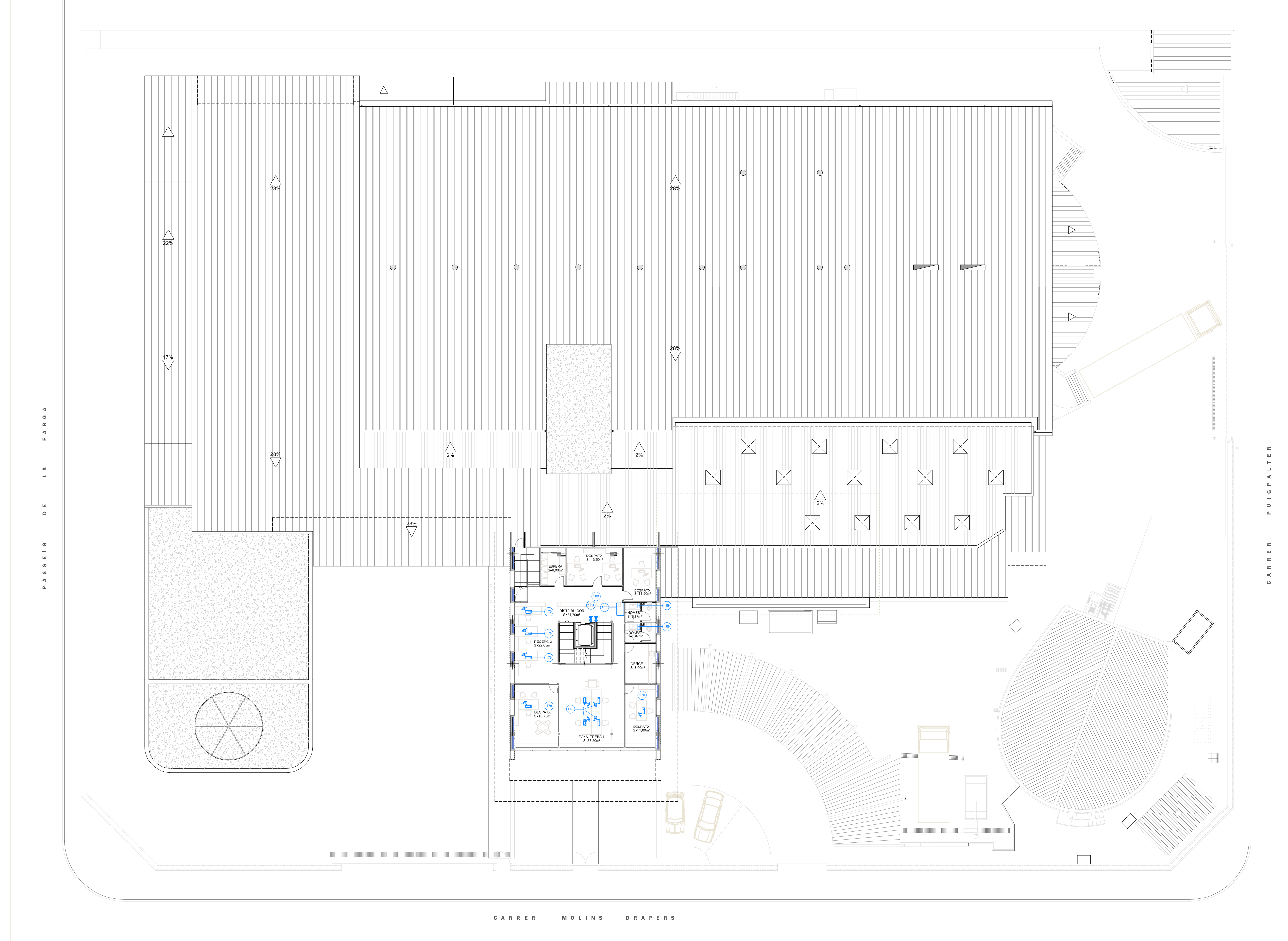
PLANTA PIS 2º E: 1/200
